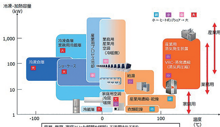
図3 ヒートポンプの利用温度帯
