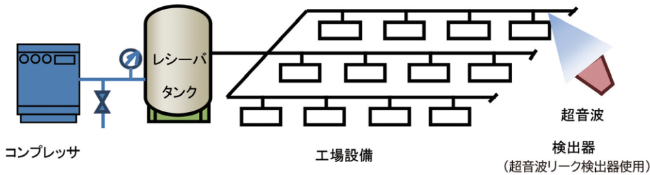
図3 圧縮空気の漏れ測定
