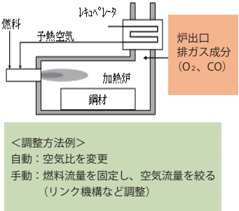
図1 工業炉（加熱炉）の空気比調整
