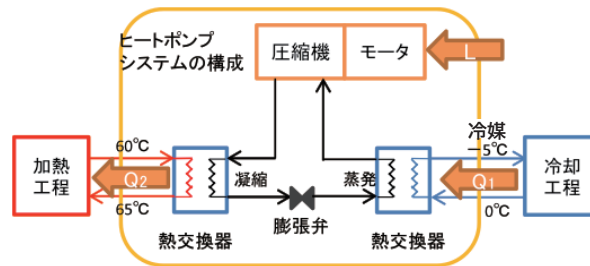
図4 ヒートポンプの概念図
